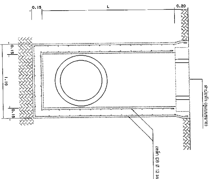
รูปตัด 2-2
