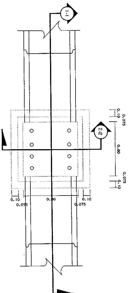
แปลนทอระบายหน้า ขนาด \varnothing 0.60 เมตร
